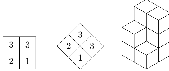
図 3: 2 \times 2 の平面分割と 3 次元 Young 図形
