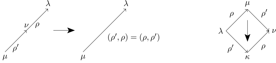
図 5: 等式 (5.5) と (5.6) の矢印による解釈
